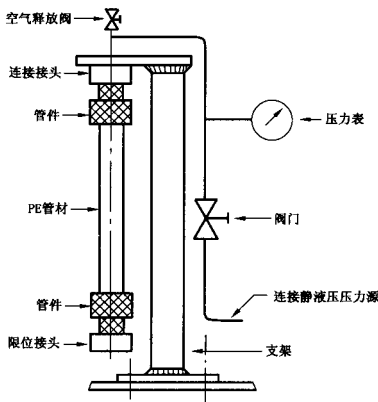
图 B.1 装置示意图
